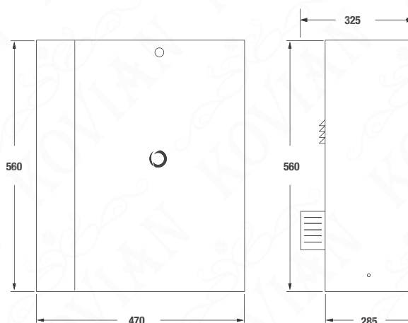
Rozměry pohonu TURBO400
